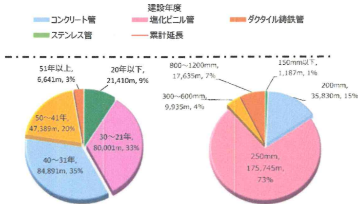
経過年数別管きょ延長 管径別管きょ延長
