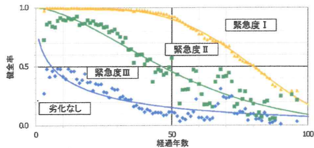
健全率予測式（鉄筋コンクリート管）
