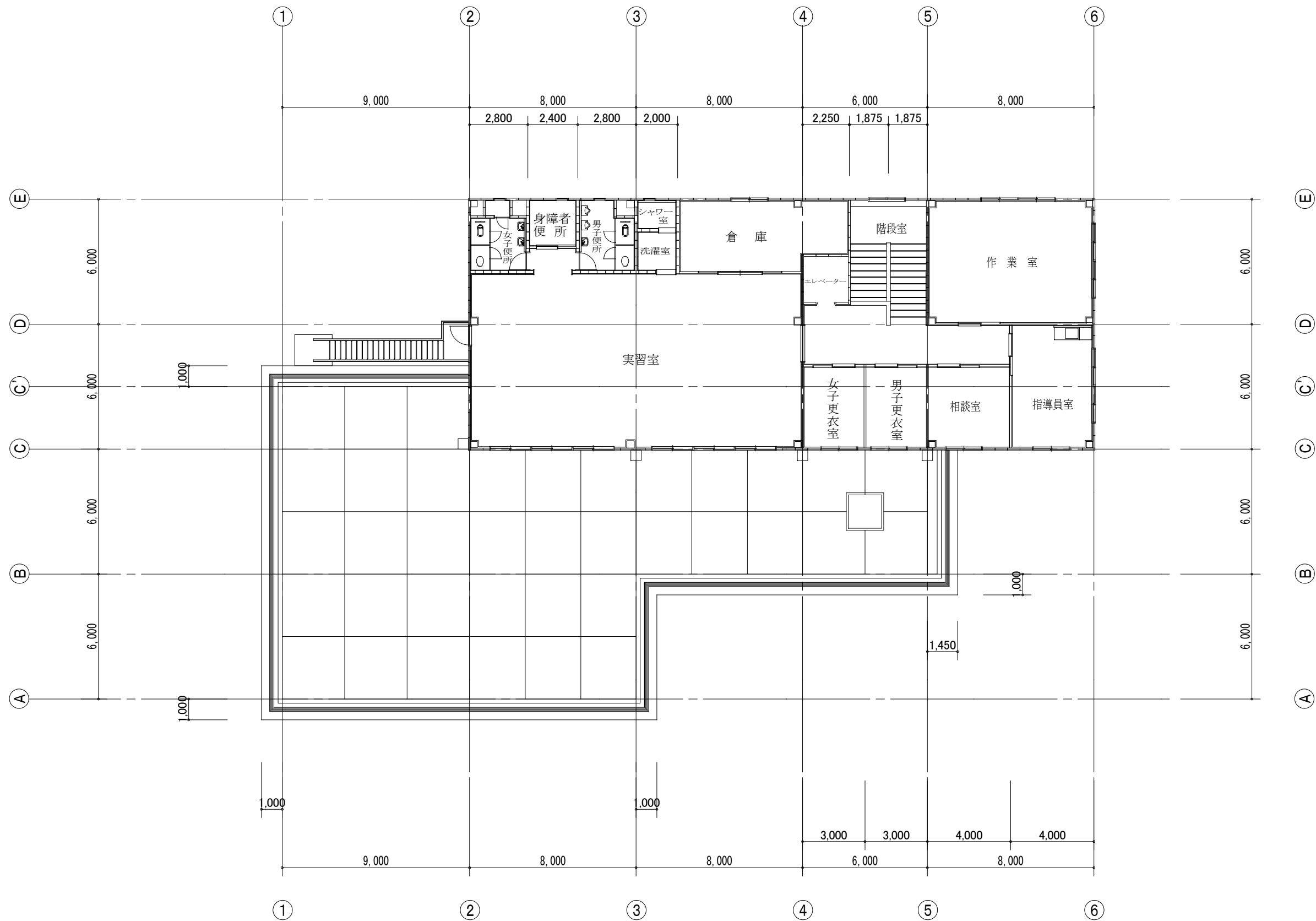
2階平面図 縮尺 1/300
