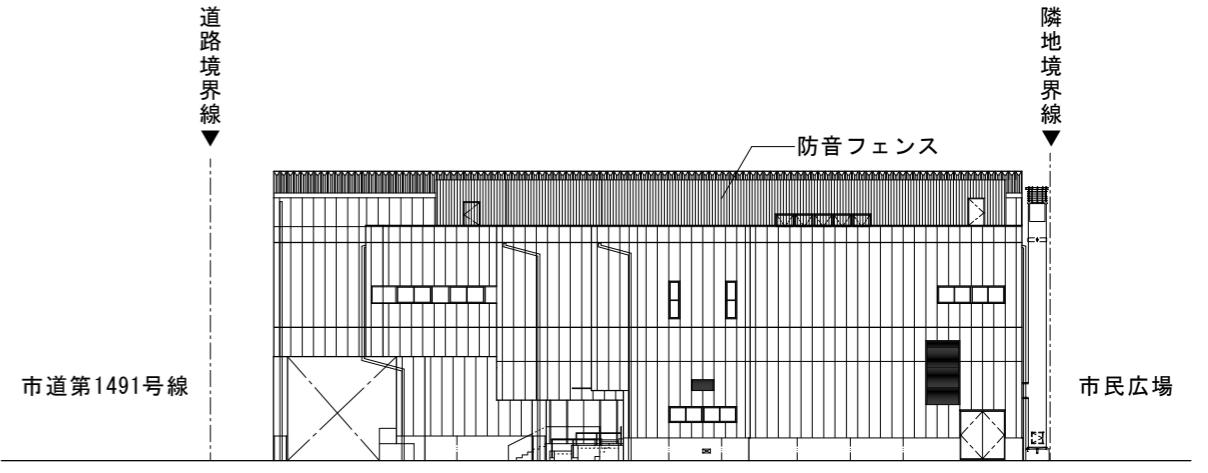
北側立面図
