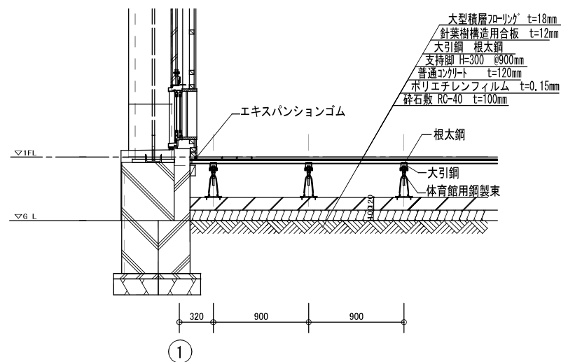
改修図
