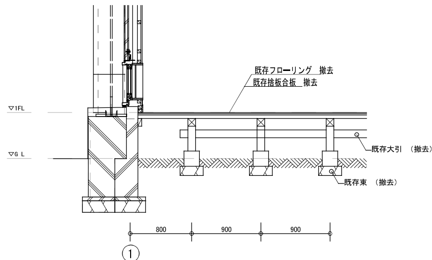
既存図
