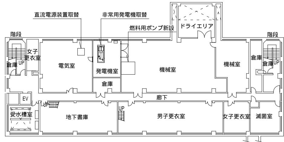
庁舎地下1階平面図
