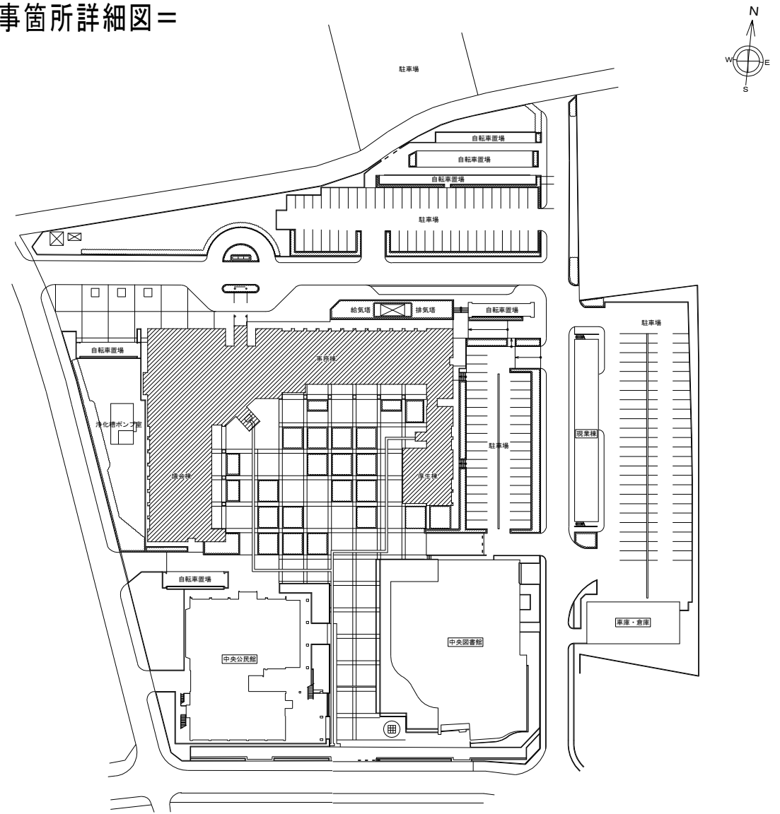
配置図 S=1/1000
