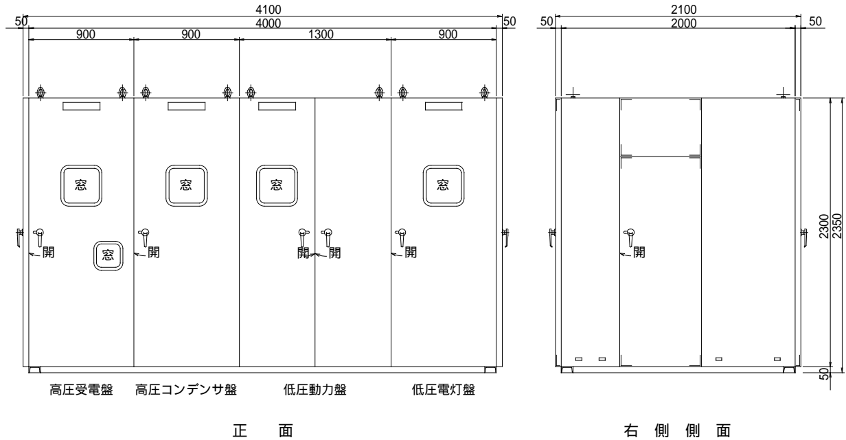
新設受変電設備 姿図
