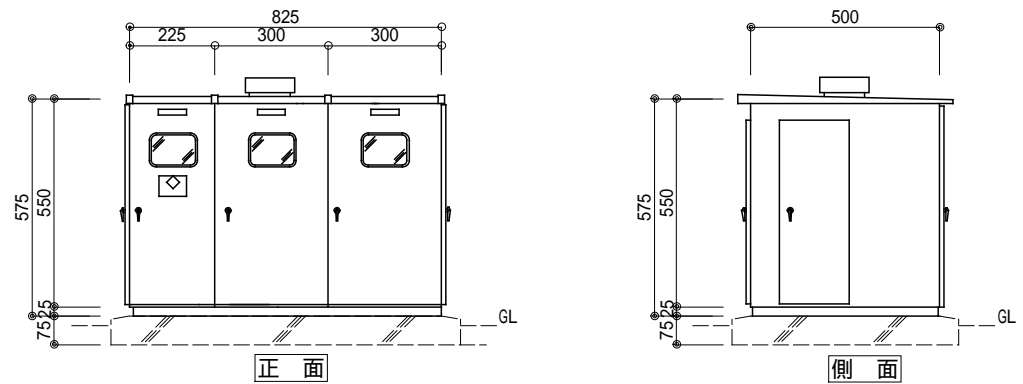
屋外型キュービクル(新設) 姿図
