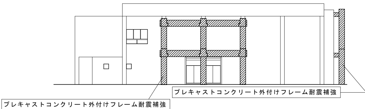
東大和市立中央公民館耐震補強工事 北側立面図
