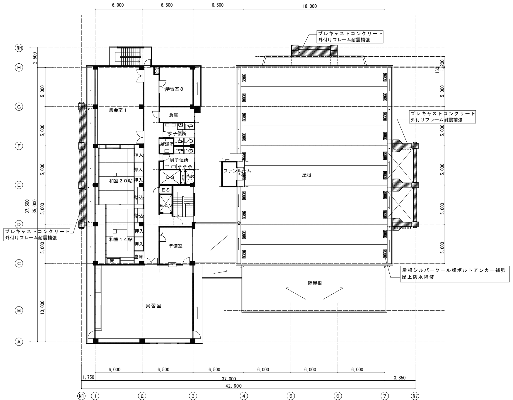
東大和市立中央公民館耐震補強工事 3階平面図
