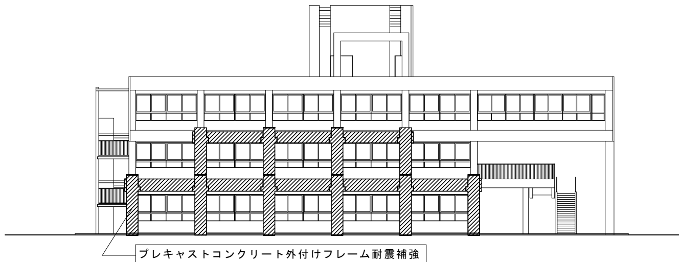
東大和市立中央公民館耐震補強工事 南側立面図
