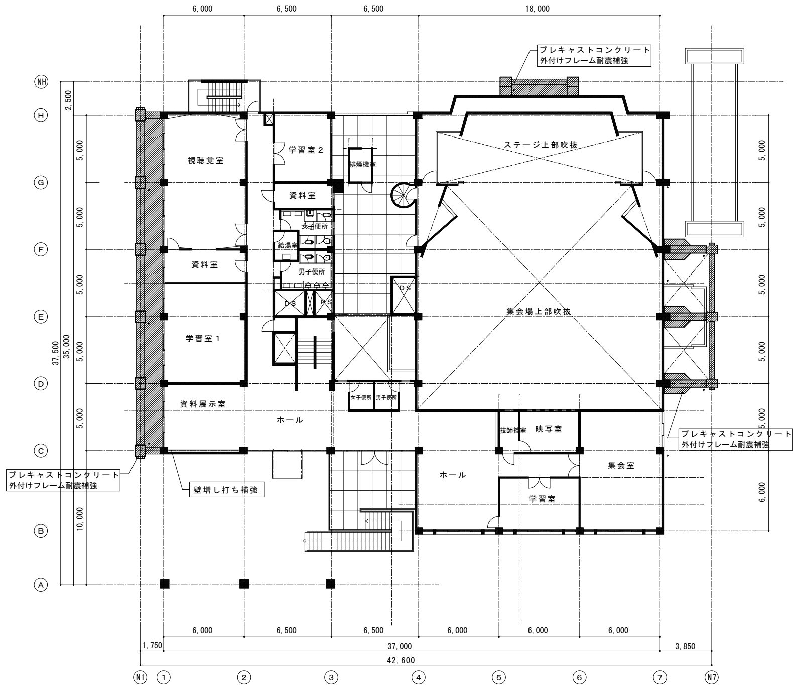
東大和市長立中央公民館耐震補強工事 2階平面図
