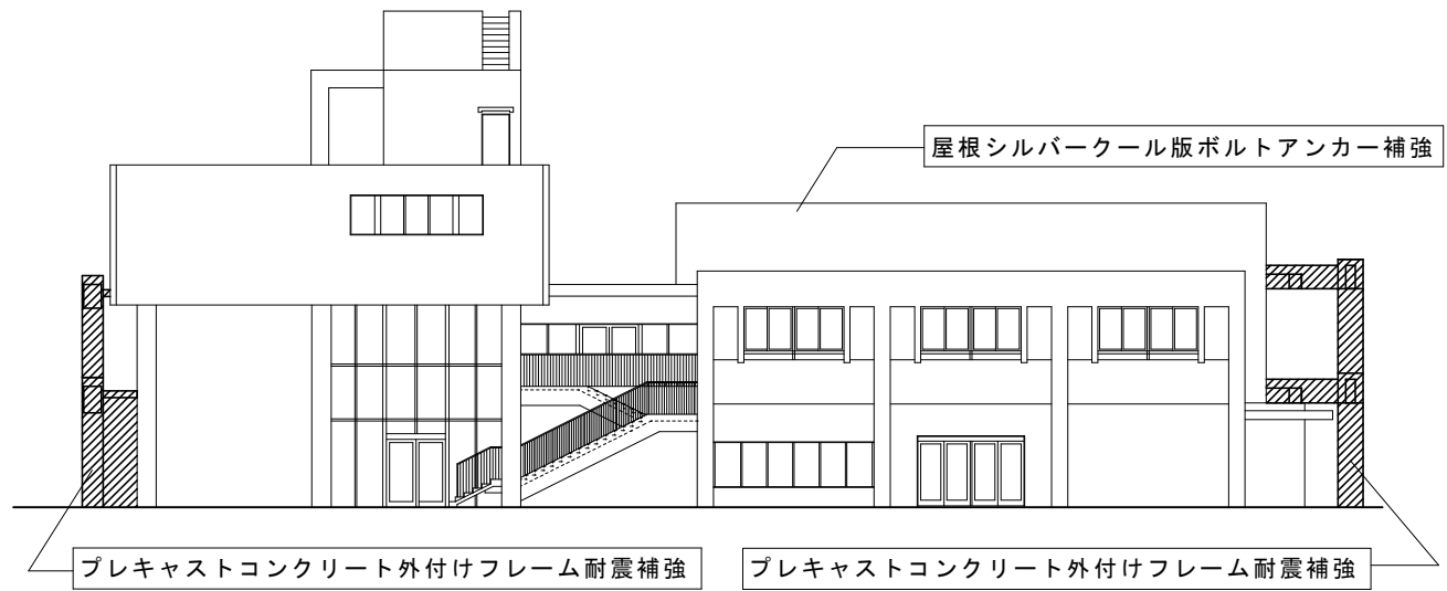
東大和市立中央公民館耐震補強工事 東側立面図
