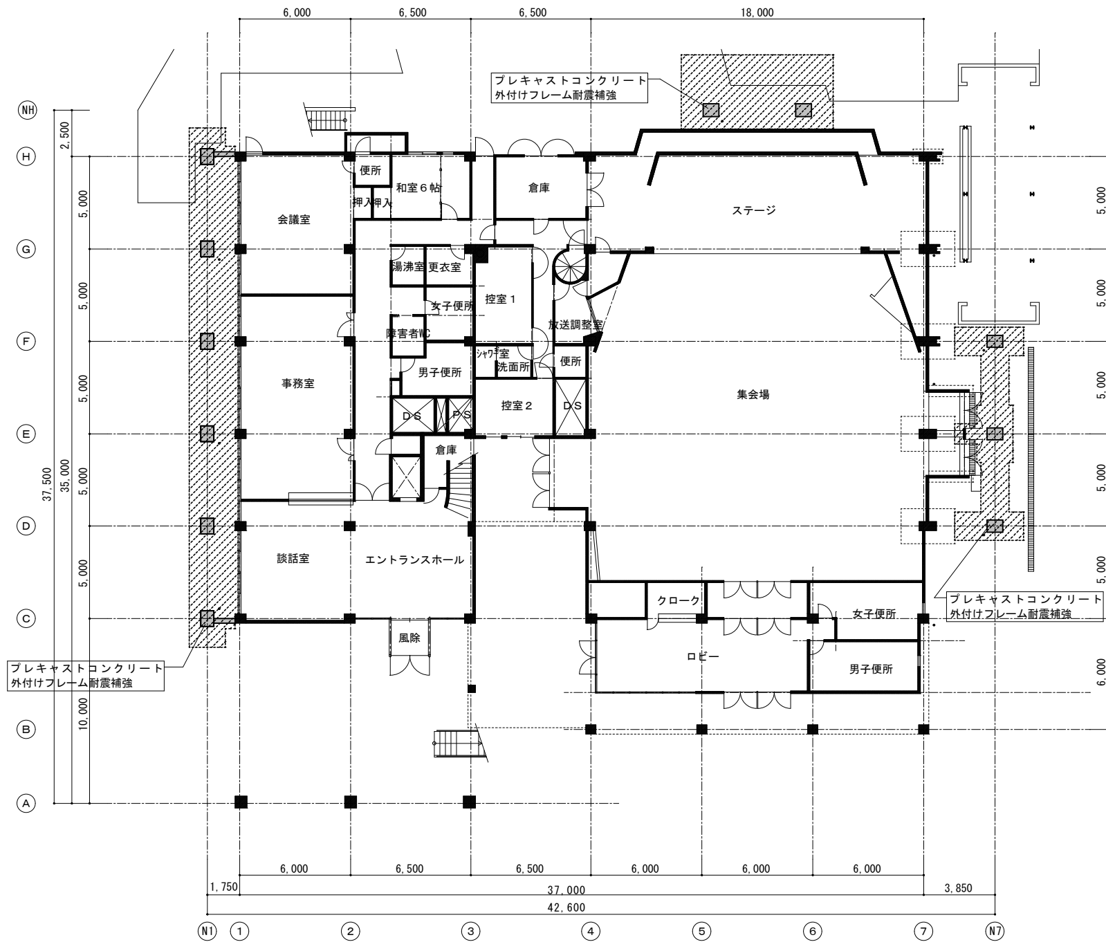
東大和市立中央公民館耐震補強工事 1階平面図
