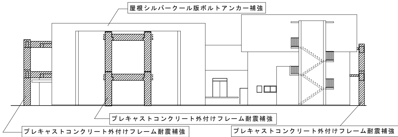
東大和市立中央公民館耐震補強工事 西側立面図
