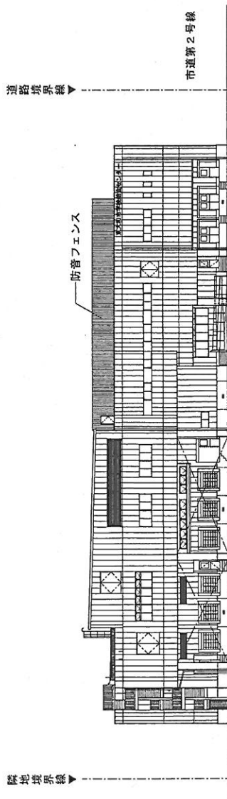
東側立面図
