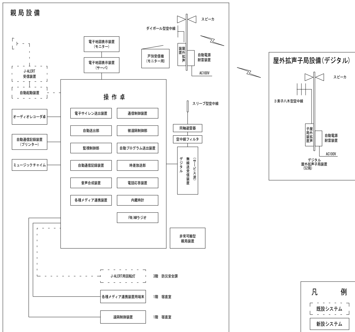
東大和市防災行政無線システム構成図(デジタル化完了時)
