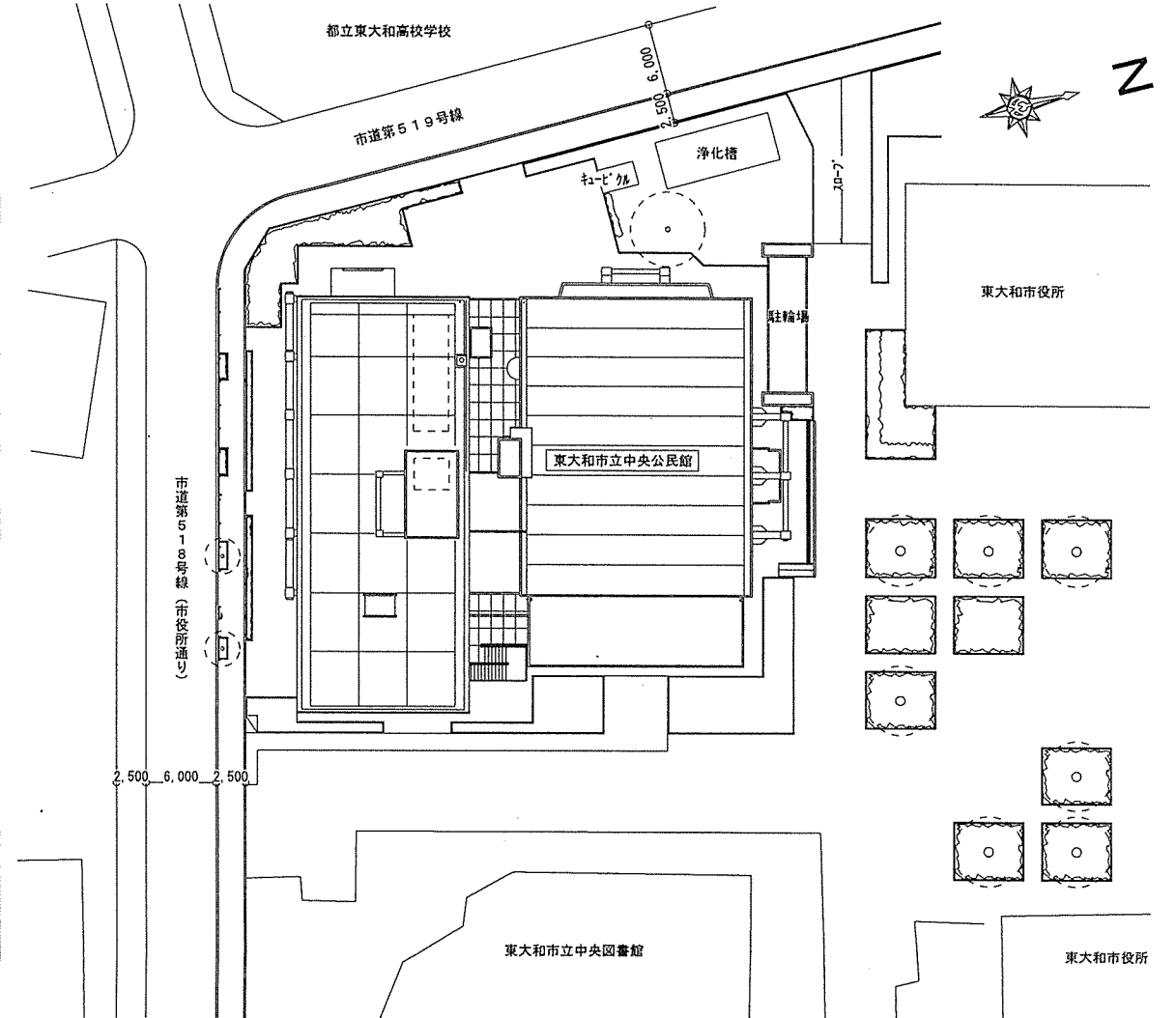
東大和市立中央公民館現況配置図 S=1:600
