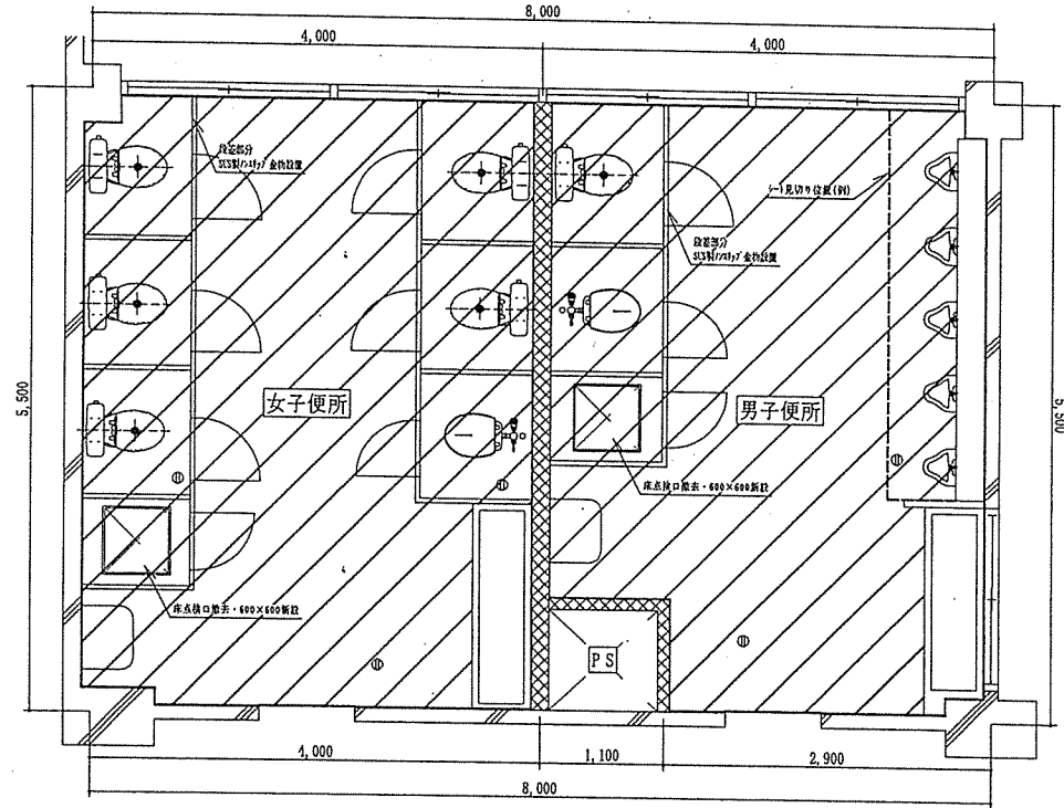
1階東側トイレ改修平面図 S=1/50
