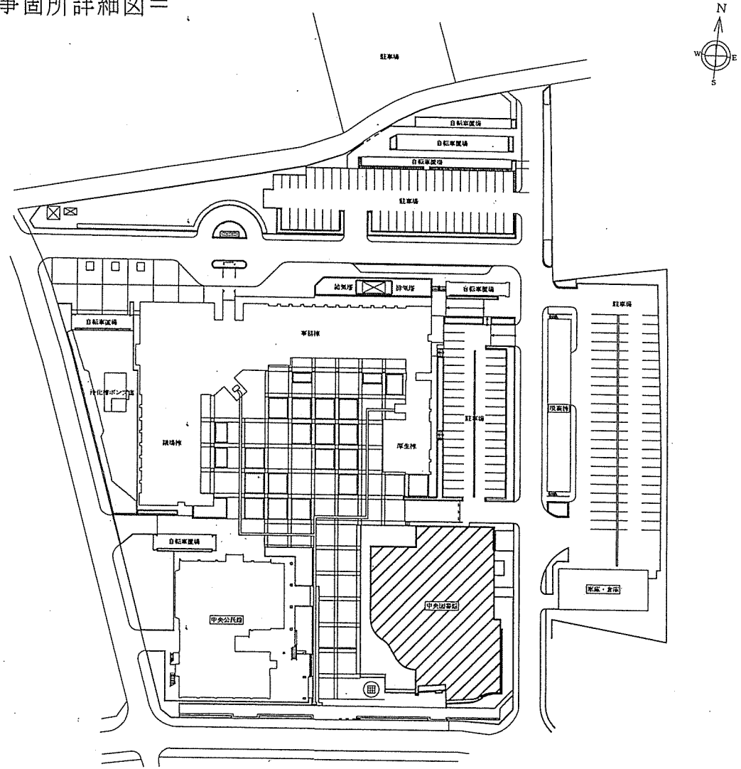
配置図 S=1/1000
