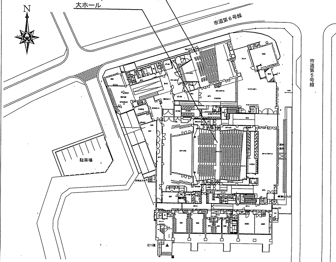
市民会館現況配置図 S=1:1000
