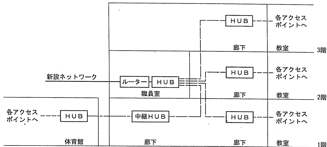
各小学校通信系統図
