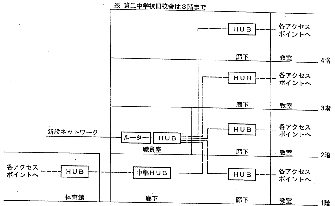
各中学校通信系統図
