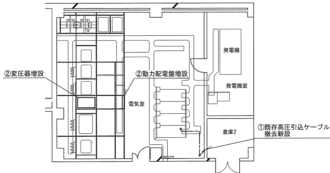
地下電気室平面図 1/150
