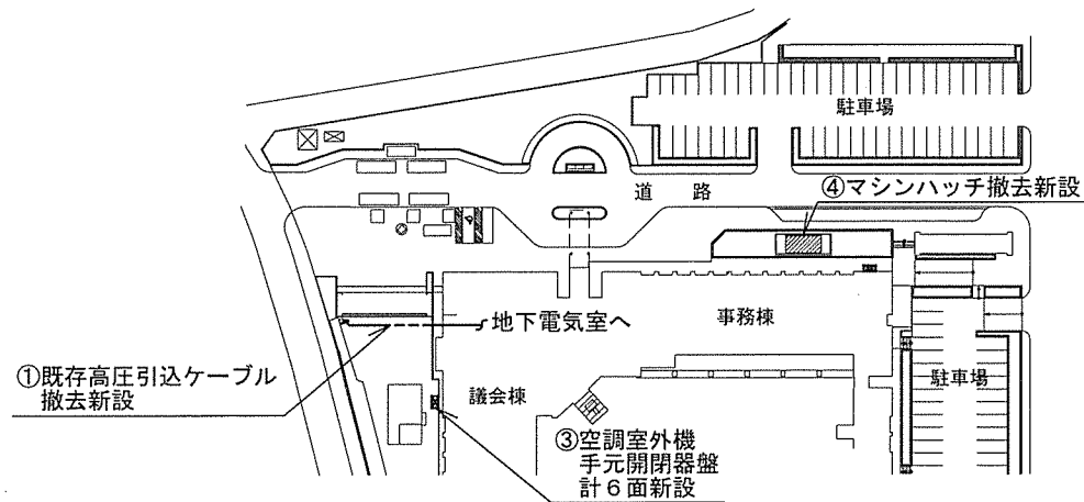
庁舎北側配置図 1/1500
