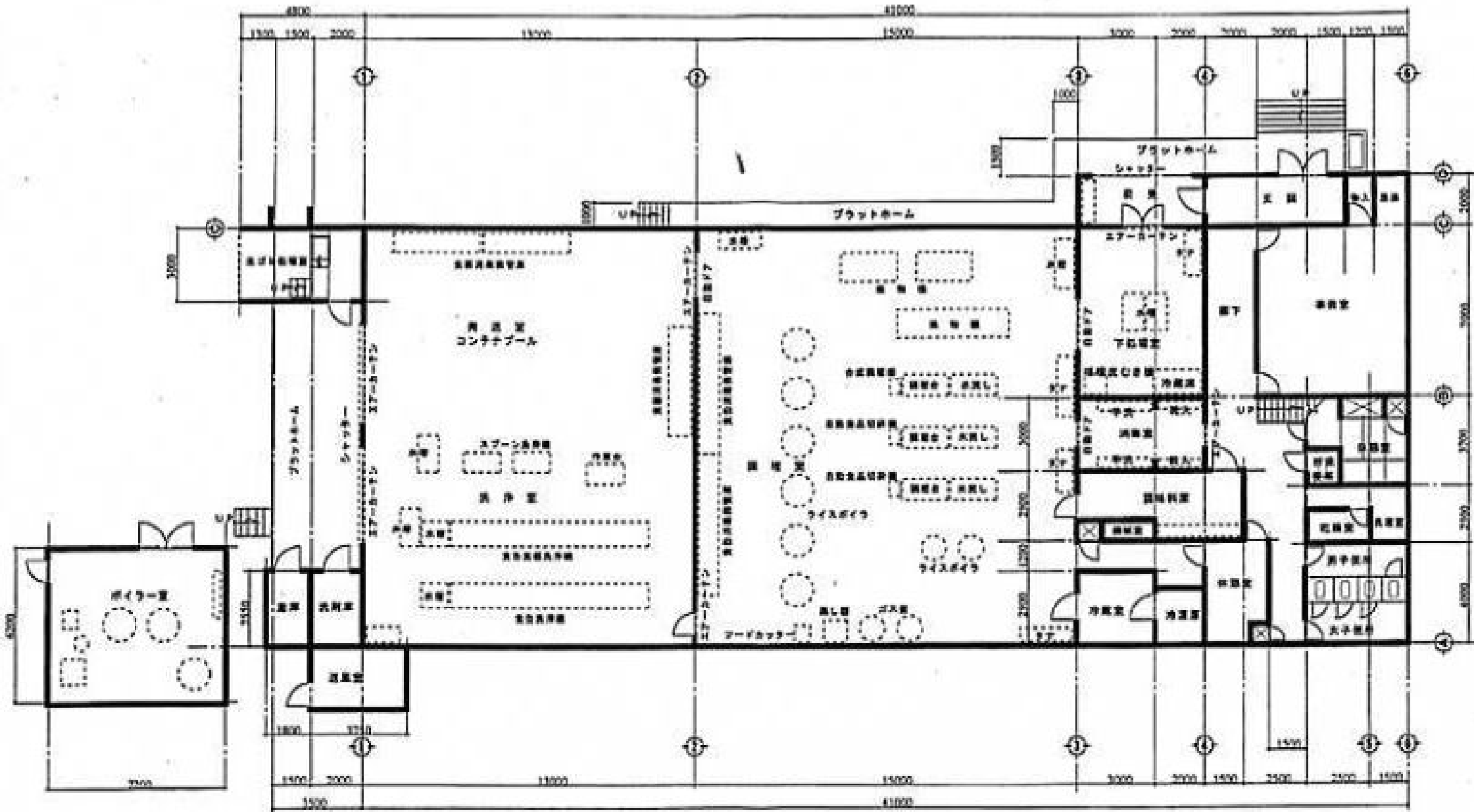
第二給食センター 1階平面図 1/150
