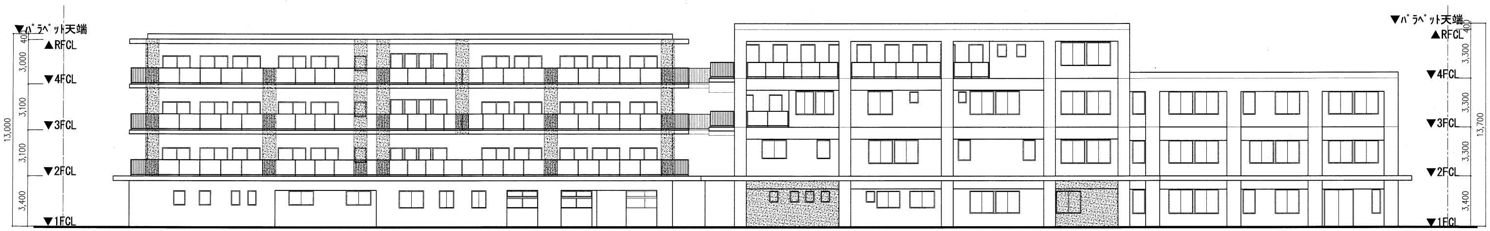
南側立面図
