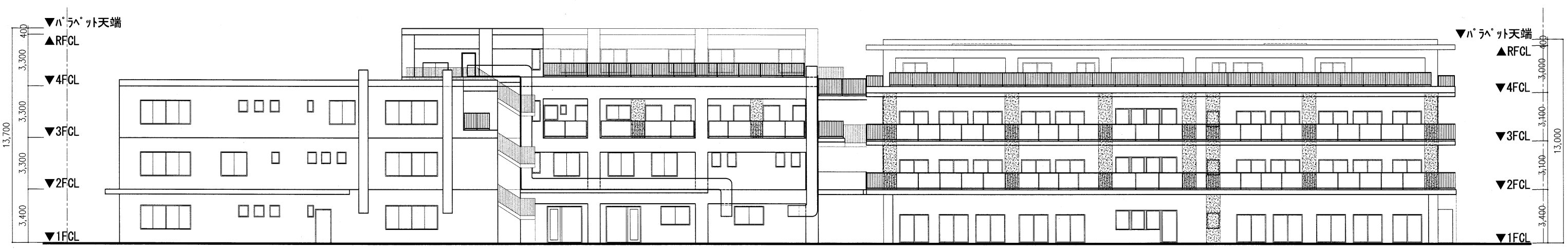
北側立面図
